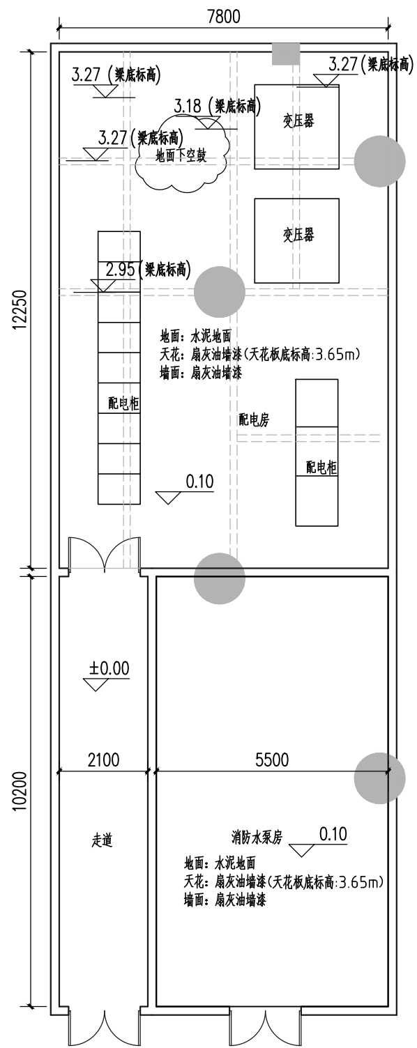
配电房、水泵房原始平面图 1:100
