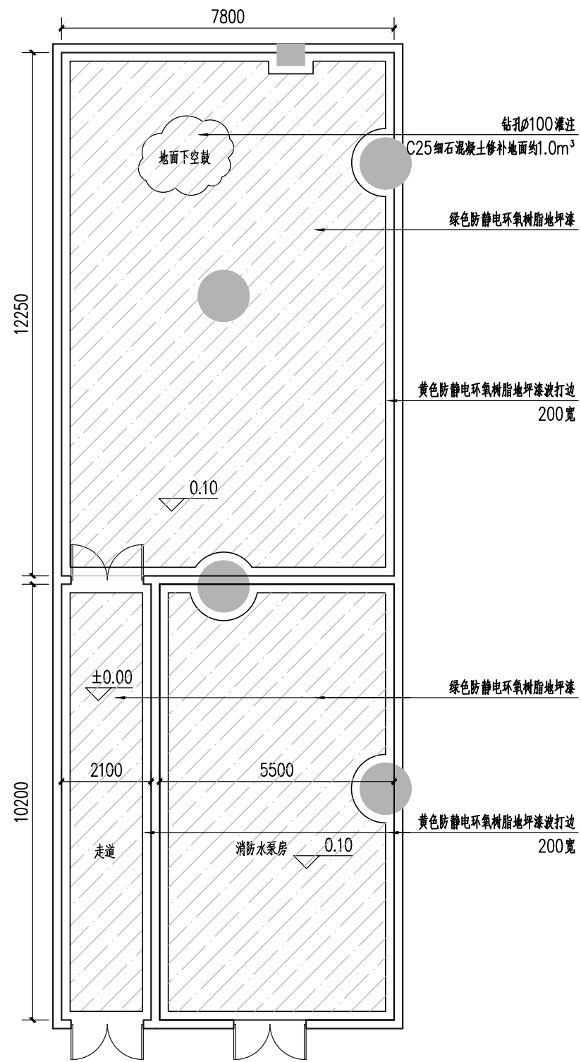
配电房、水泵房地面铺装平面图 1:100
