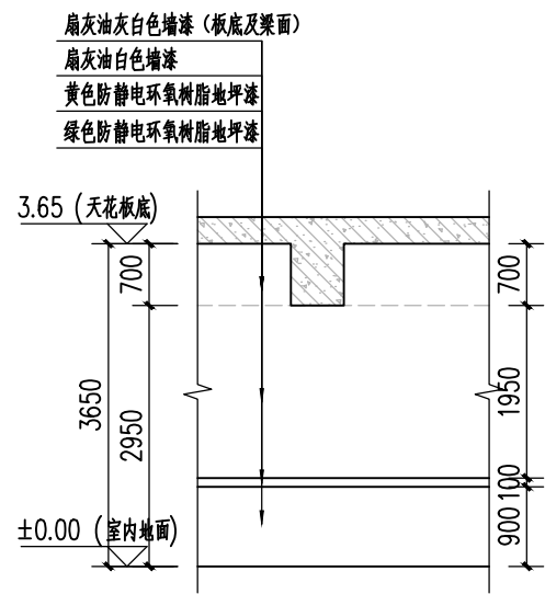
墙面做法大样图
