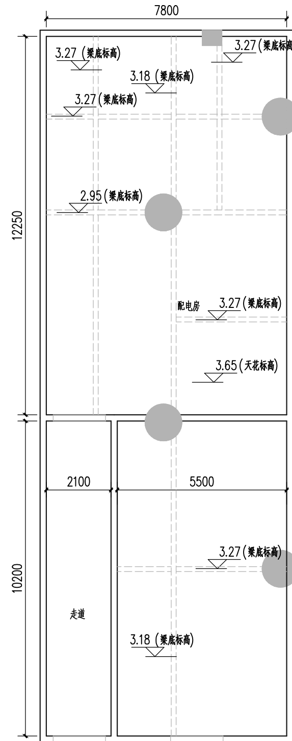
配电房、水泵房天花平面图 1:100
