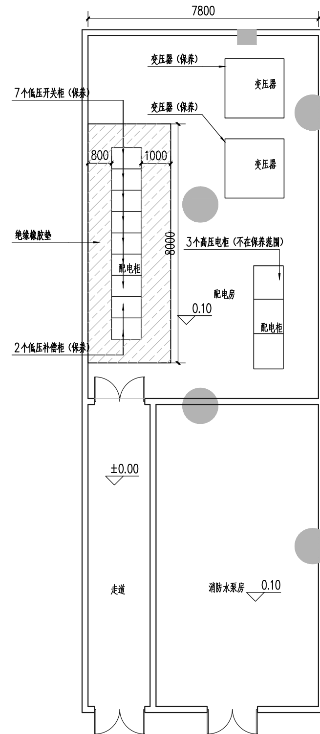
配电房配电柜保养图 1:100
