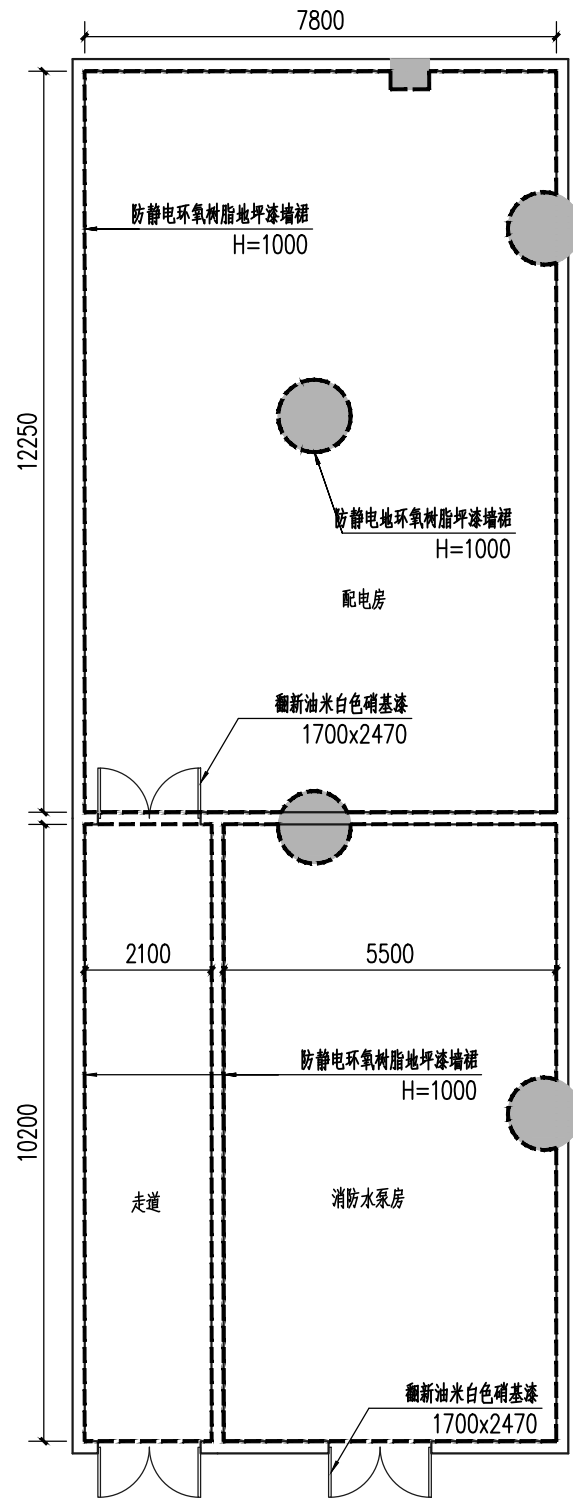
配电房、水泵房墙面平面图 1:100
