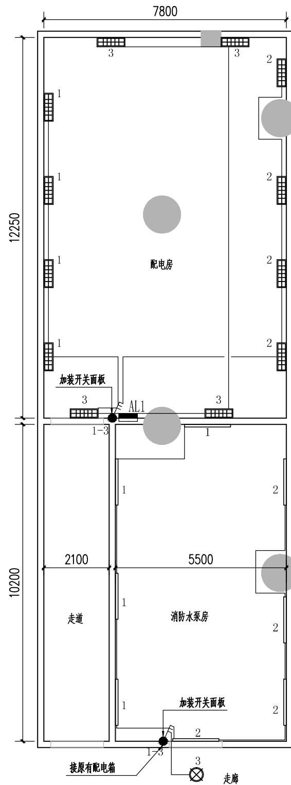
配电房、水泵房照明及灯控图 1:100
